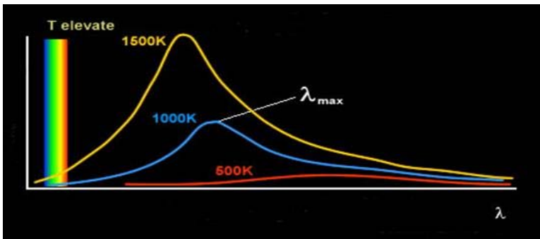
Spettro di emissione di un corpo nero
